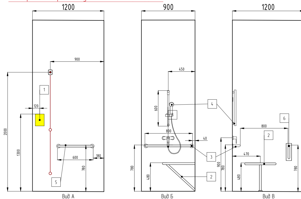
Развертки открытой душевой кабины 900x1200
