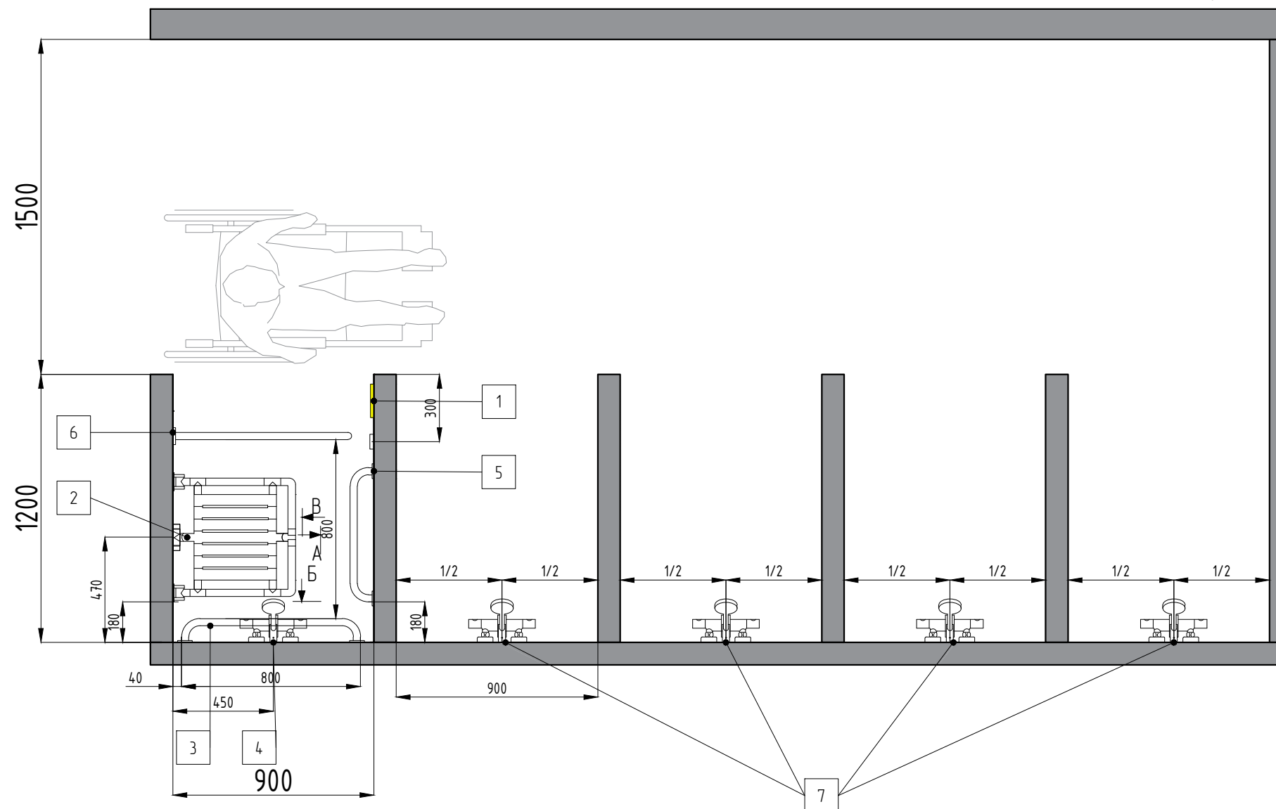
Развертки открытой душевой кабины 900x1200
